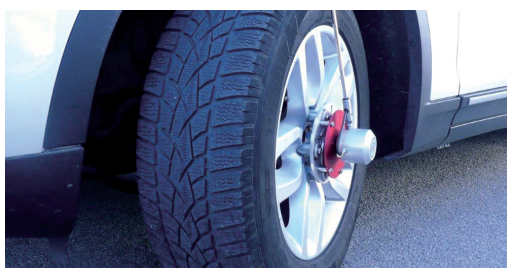
Capteur de déplacement avec Peiseler Plaque de montage monté sur une roue de voiture
